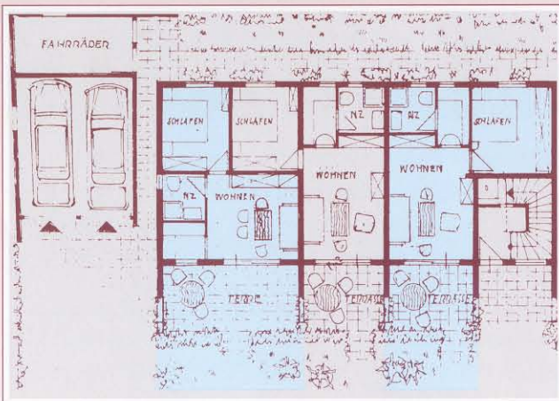
Grundriß der drei Komfort-Appartements im Nebenhaus
